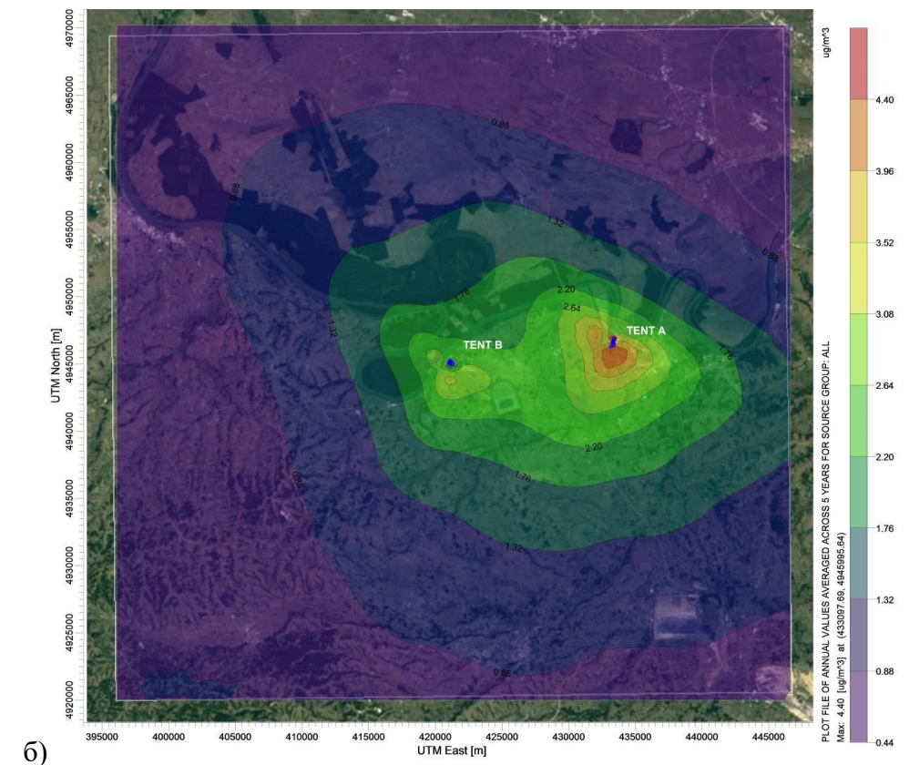
Слика 3.1. Приказ резултата моделирања распрострања сумпорних оксида приказаних као \text{SO}_2 , за период усредњавања од једне календарске године (а- тренутно стање, б-стање након 01.01.2028. године)
