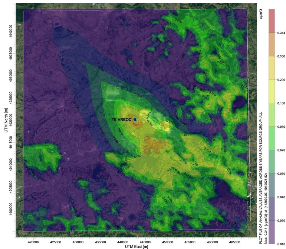
Слика 3.8. Приказ резултата моделирања распрострања азотних оксида приказаних као \text{NO}_2 , за период усредњавања од једне календарске године (постојеће стање)
