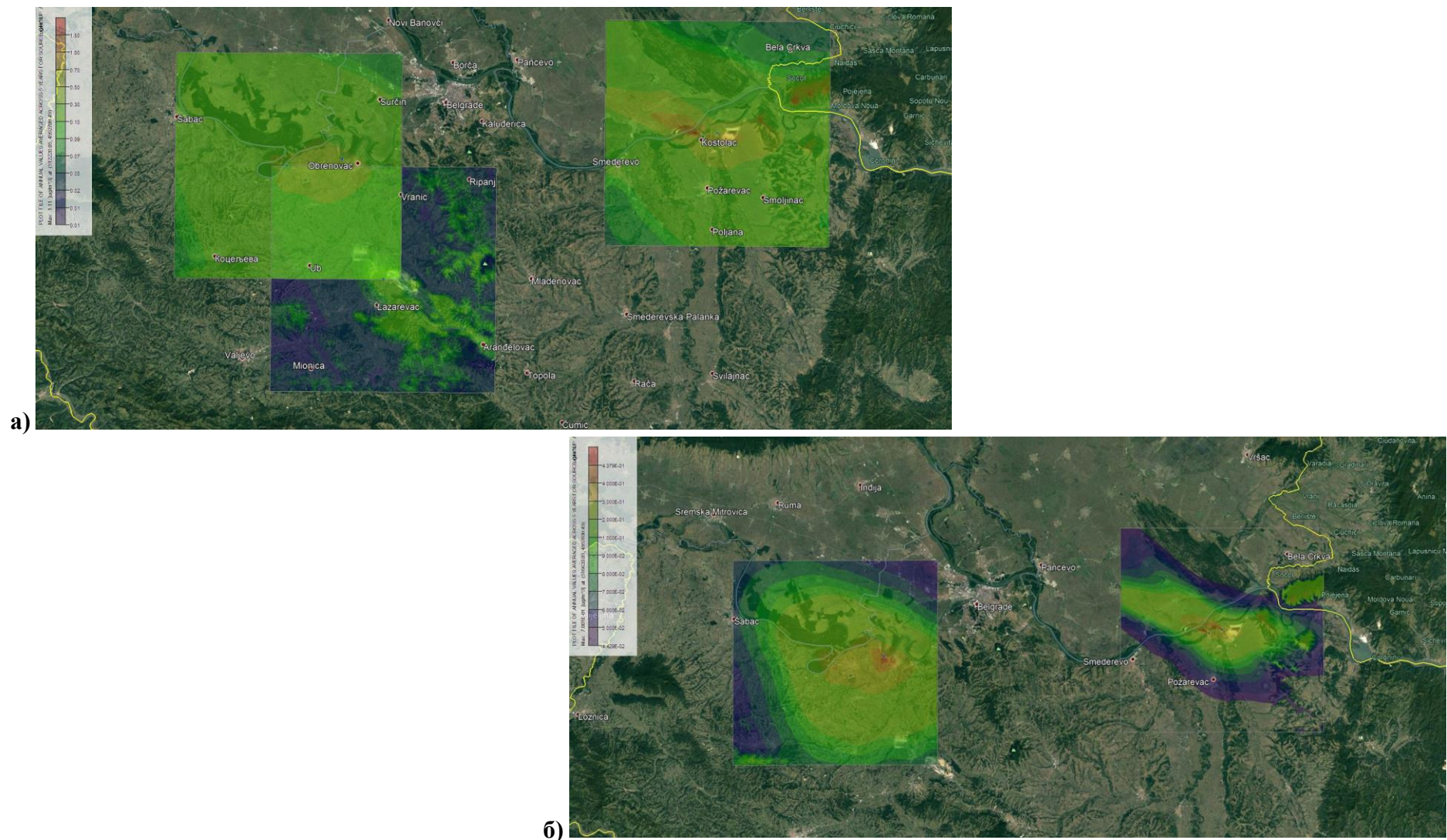
Слика 3.12. Приказ резултата моделирања распрострањања PM_{10} , за период усредњавања од једне календарске године(а- тренутно стање, б-стање након 01.01.2028. године)
