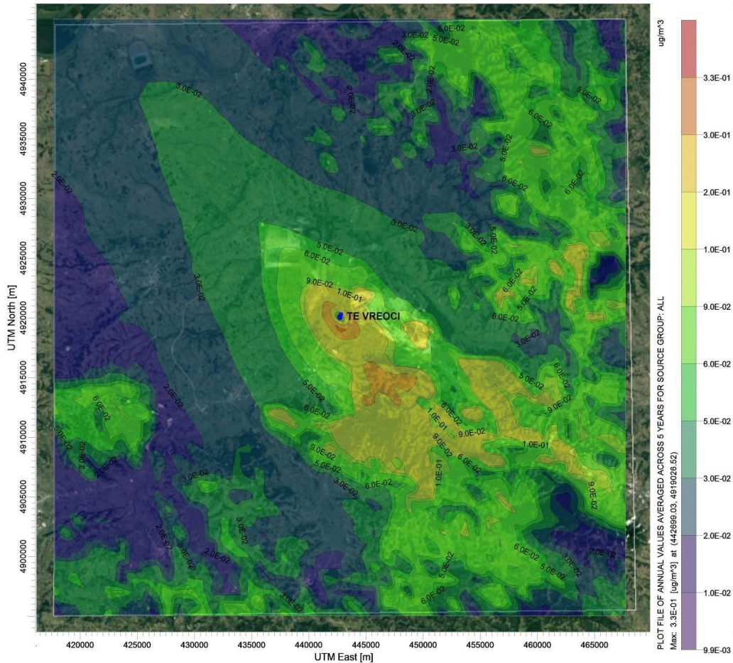
Слика 3.9. Приказ резултата моделирања распрострања PM10 за период усредњавања од једне календарске године (постојеће стање)
