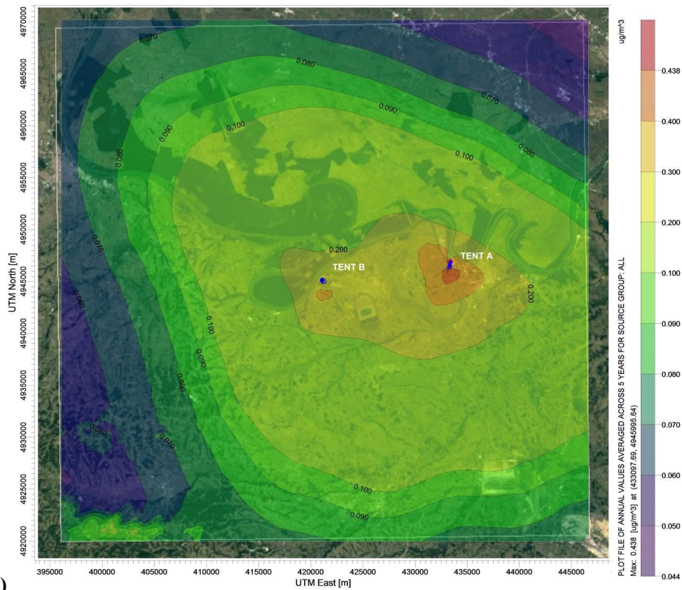
Слика 3.3. Приказ резултата моделирања распрострања PM10 за период усредњавања од једне календарске године (а- тренутно стање, б-стање након 01.01.2028. године)
