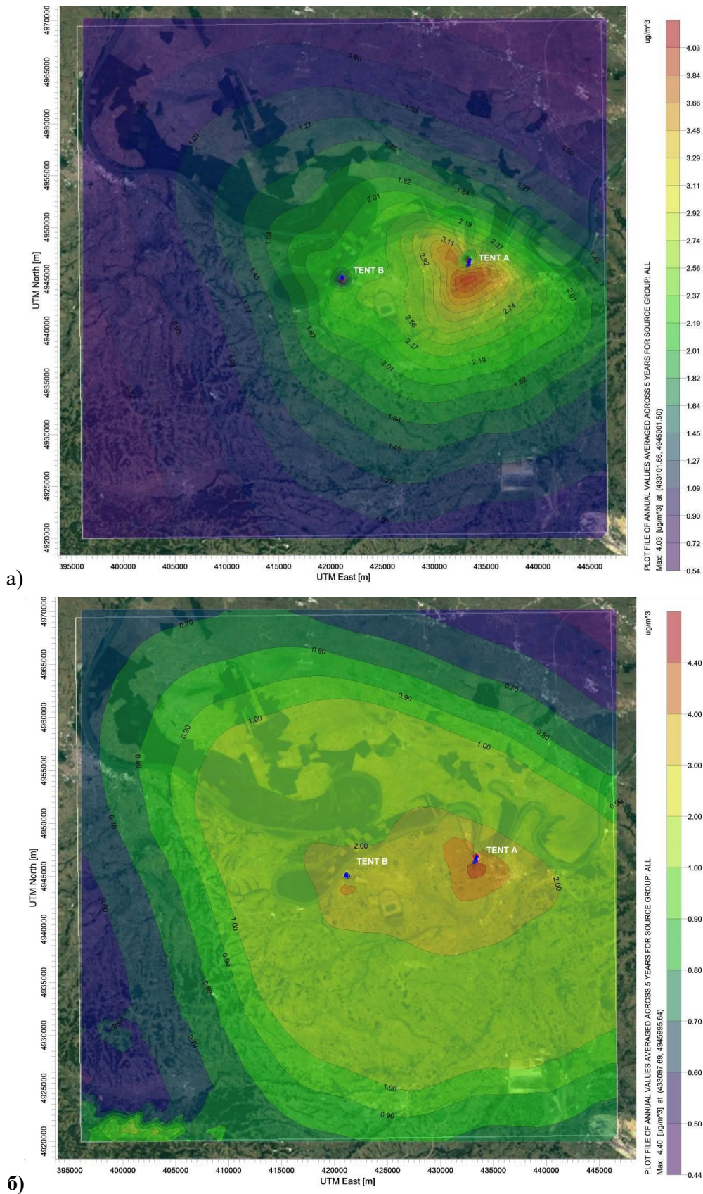
Слика 3.2. Приказ резултата моделирања распрострања азотних оксида приказаних као \text{NO}_2 , за период усредњавања од једне календарске године (а- тренутно стање, б-стање након 01.01.2028. године)
