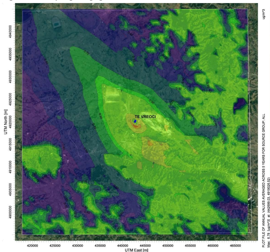
Слика 3.7. Приказ резултата моделирања распрострања сумпорних оксида приказаних као \text{SO}_2 , за период усредњавања од једне календарске године (постојеће стање)
