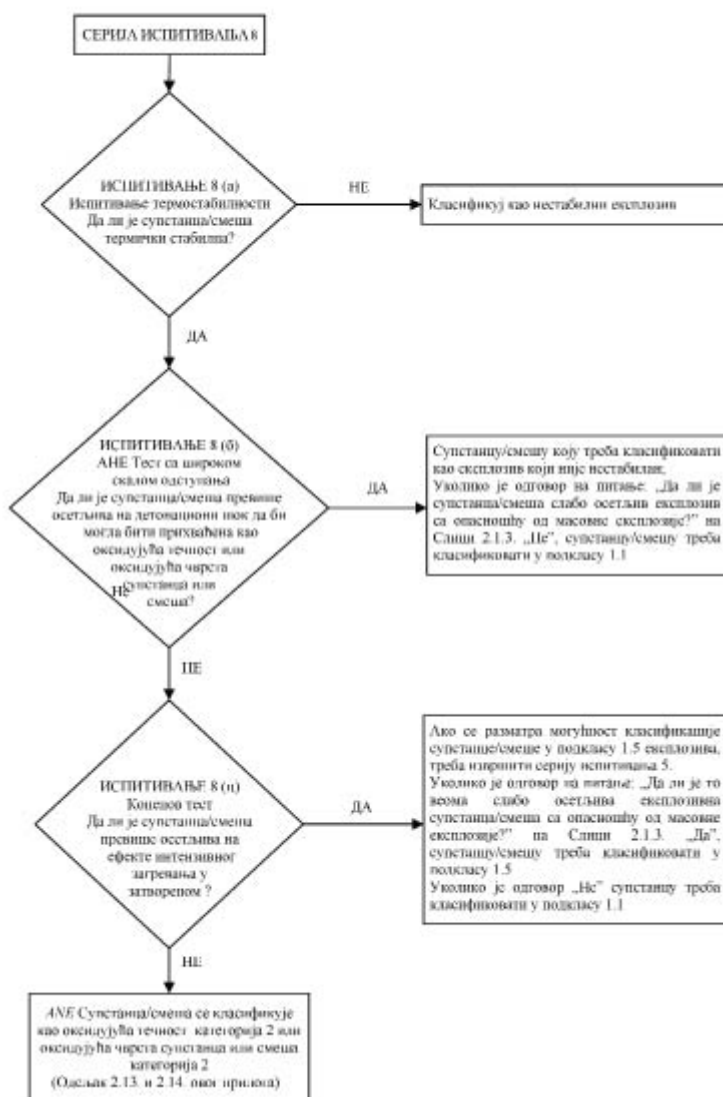
Слика 2.1.4. Поступак класификације амонијум-нитратних емулзија, раствора и гелова (ANE)
