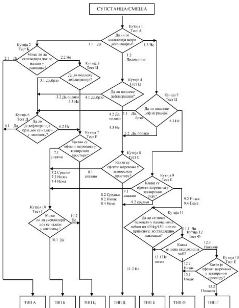
Слика 2.8.1. Самореактивне супстанце и смеше
