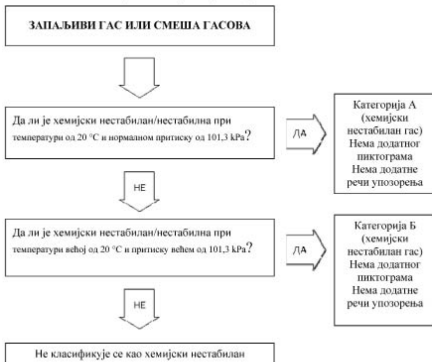
Слика 2.2.2. Поступак класификације хемијски нестабилних гасова
