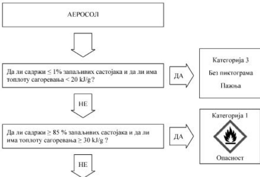
Слика 2.3.1(1) Аеросоли
