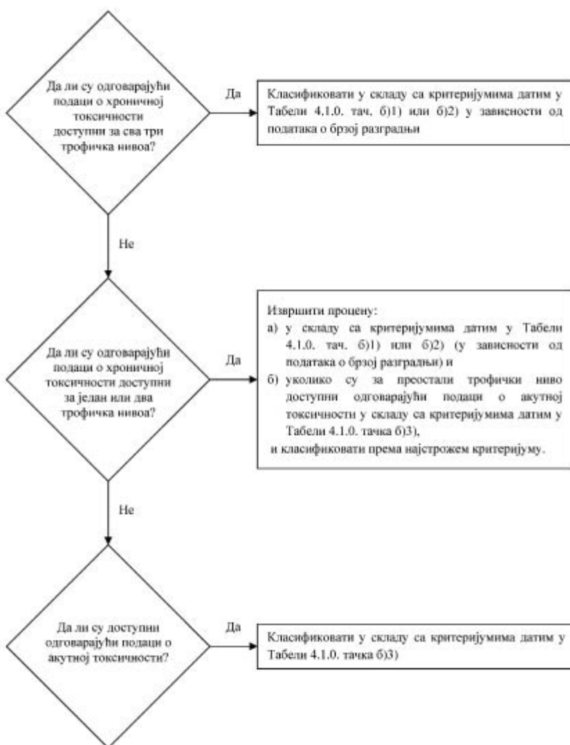
Слика 4.1.1. Поступак класификације супстанци у категорије дуготрајне опасности по водену животну средину
