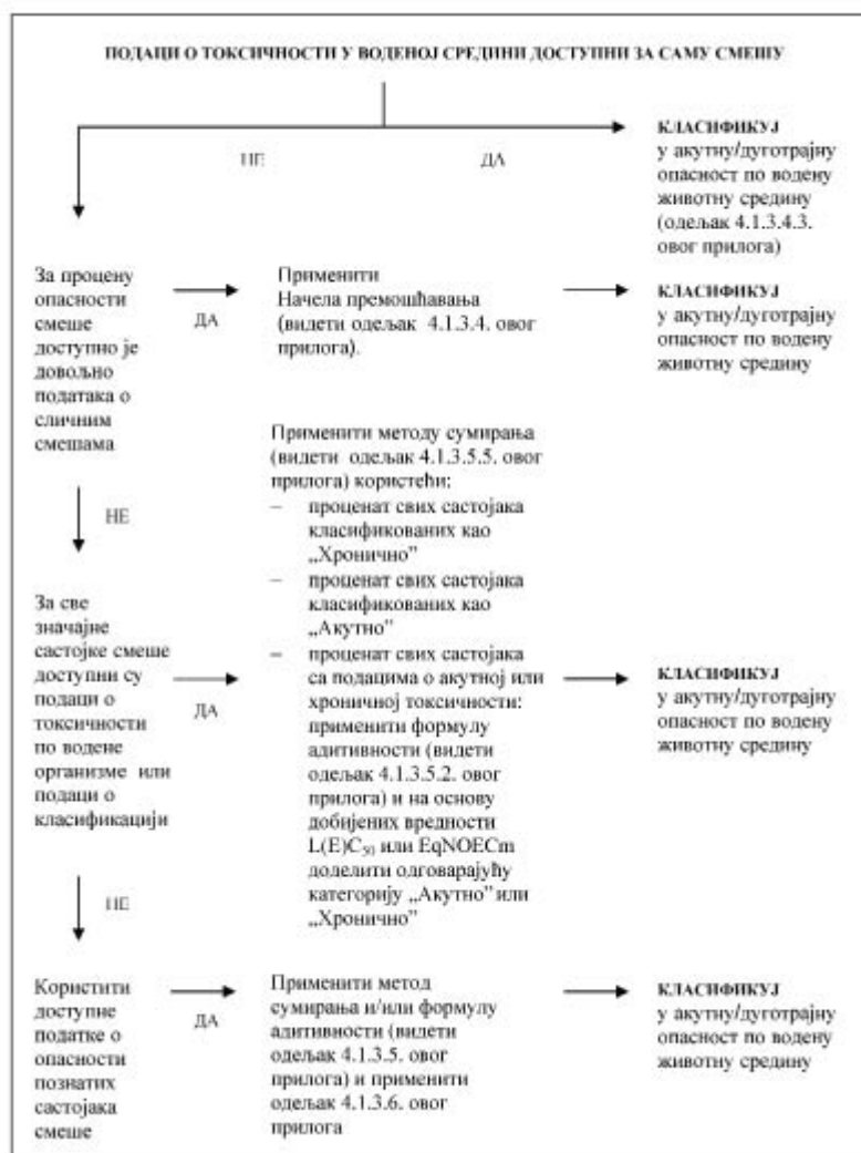
Слика 4.1.2. Вишестепени приступ класификацији смеша у односу на акутну и дуготрајну опасност по водену животну средину
