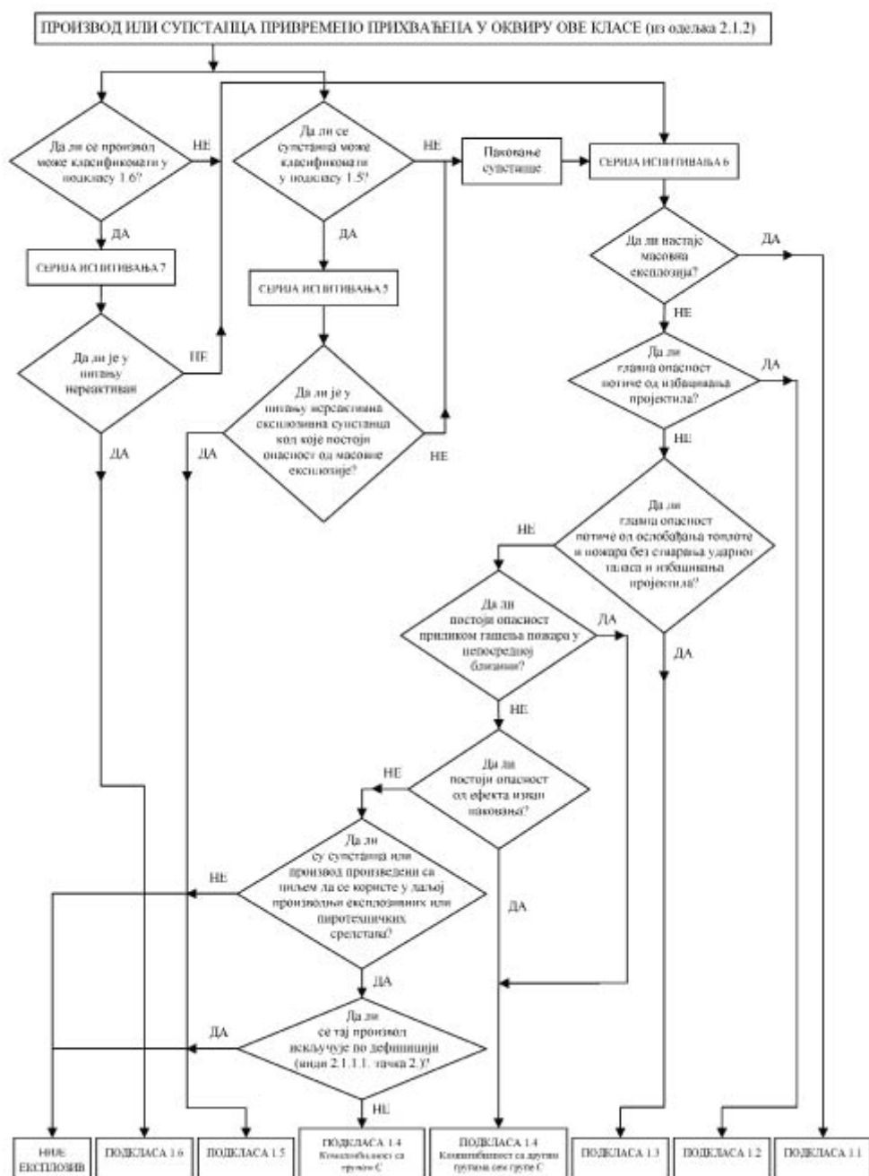
Слика 2.1.3. Поступак класификације у једну од подкласа класе експлозива (Класа 1 за транспорт опасног терета)
