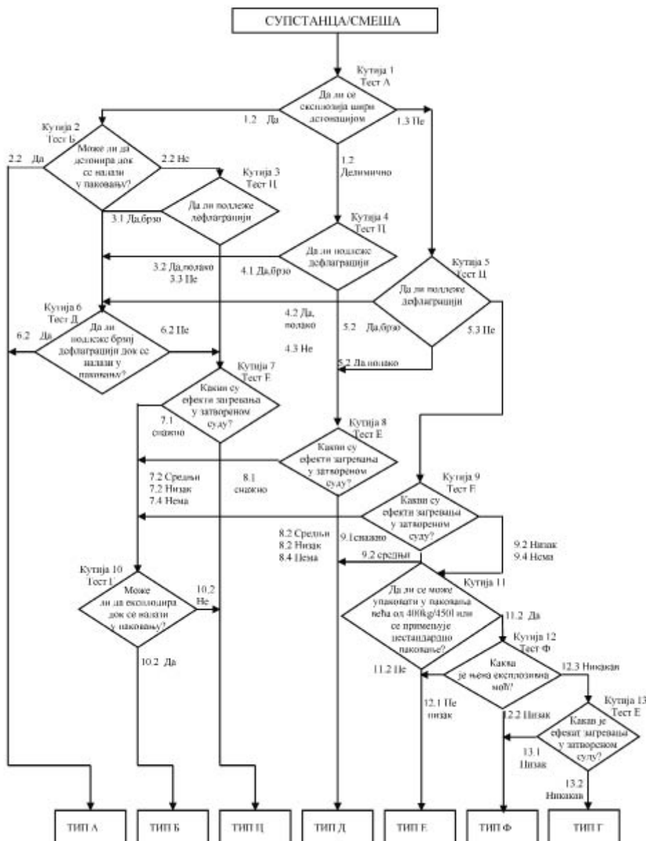
Слика 2.15.1. Органски пероксиди
