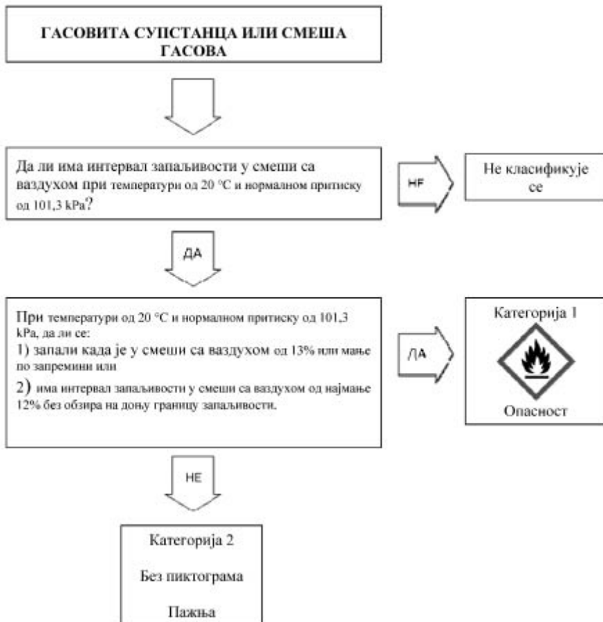
Слика 2.2.1. Поступак класификације запаљивих гасова
