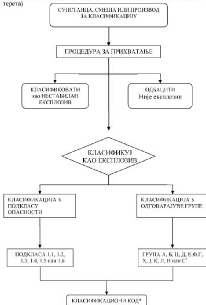
Слика 2.1.1. Општа шема поступка за класификацију супстанце, смеше или производа у једну од подкласа експлозива (Класа 1 за транспорт опасног терета)
