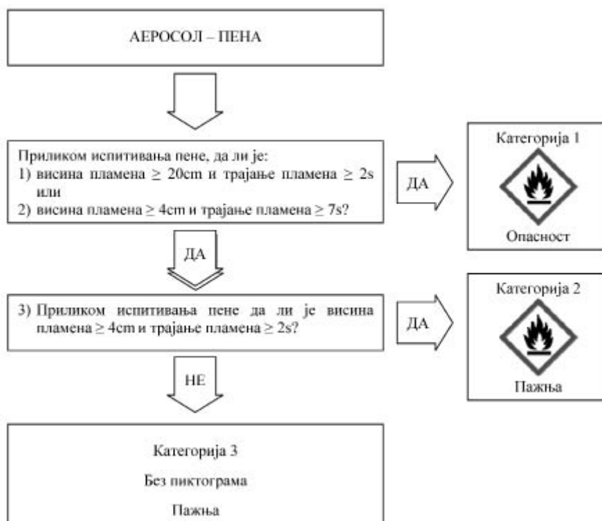
Слика 2.3.1(3) Аеросол – пена
