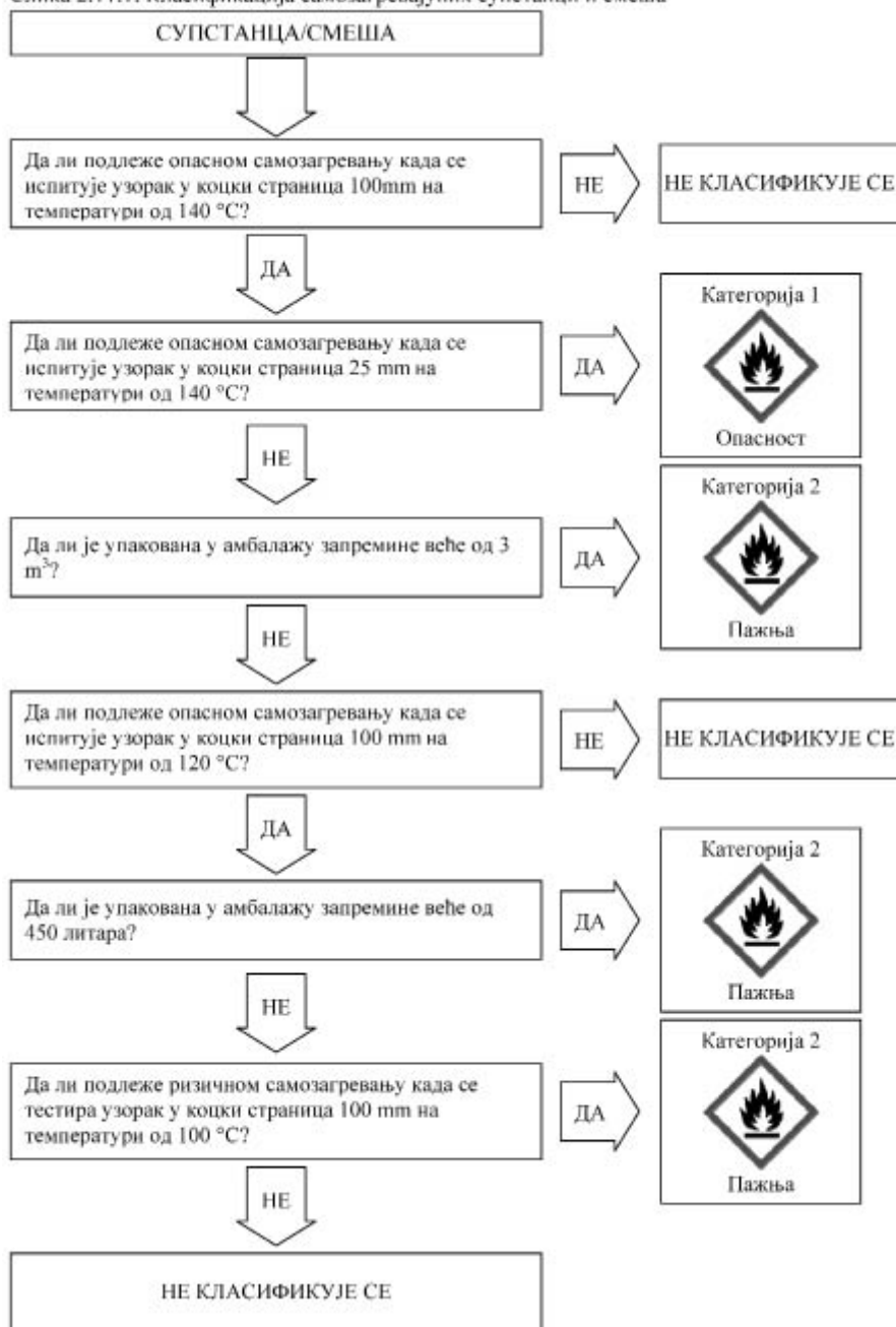
Слика 2.11.1. Класификација самозагревајућих супстанци и смеша
