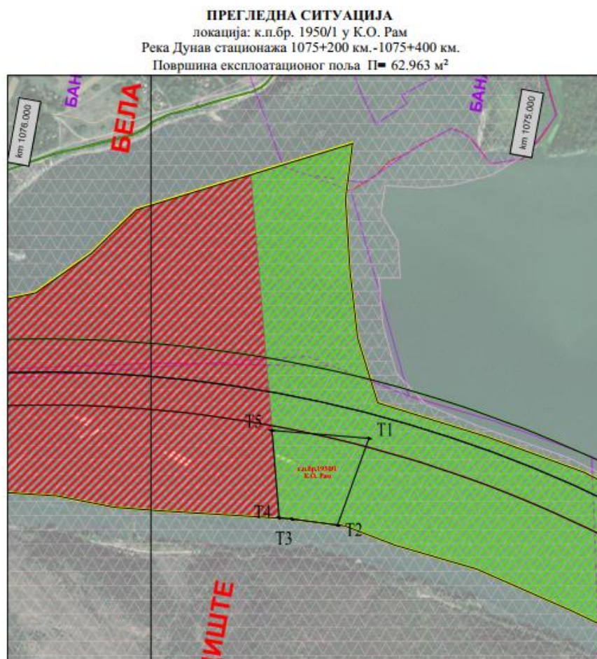
Координате дна кинете експлоатационог поља у ГК 7. зони
