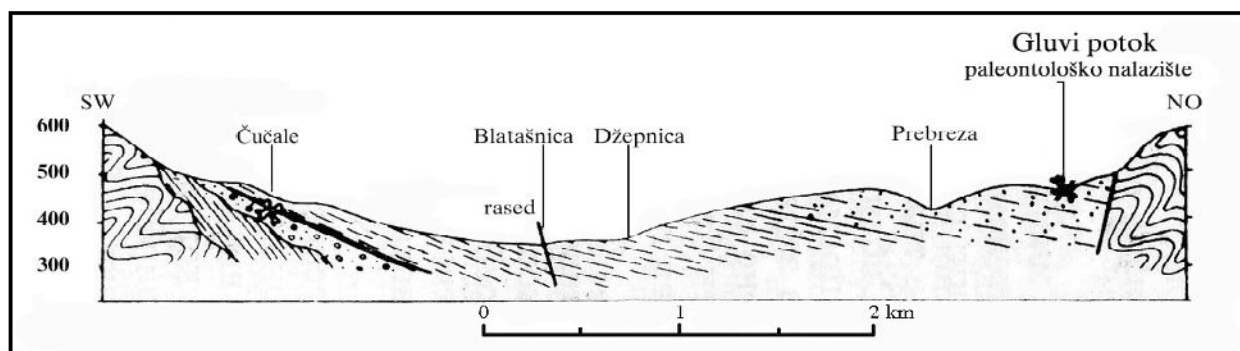
Шематски попречни геолошки профил северозападног дела Топличког басена (легенда-Литостратиграфски стуб на стр. 8) (преузето из Павловић М, 1969)
