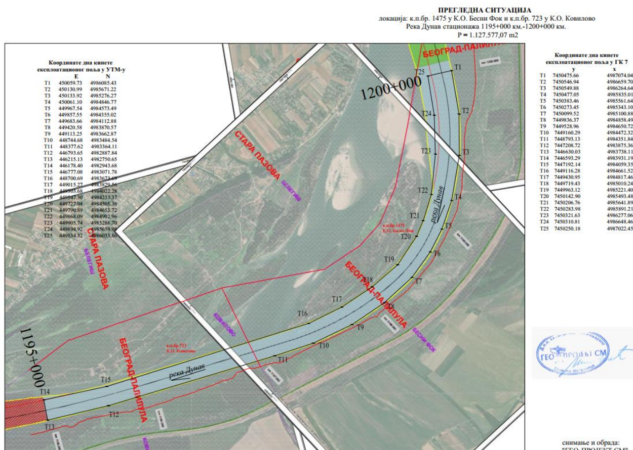
Слика -Ситуација шире локације реке Дунав (од км 1195+000 до км 1200+000)
